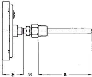
4 - Осовой монтаж
