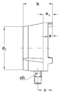
A - ПРИСОЕДИНЕНИЕ СНИЗУ
