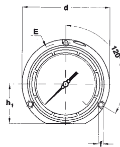
D - ПРИСОЕДИНЕНИЕ СЗАДИ, ТОЛЬКО ДЛЯ СТАНДАРТНОЙ МОДЕЛИ
