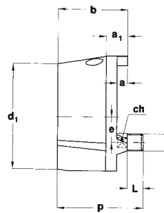
D - ПРИСОЕДИНЕНИЕ СЗАДИ, ТОЛЬКО ДЛЯ СТАНДАРТНОЙ МОДЕЛИ
