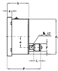
D - Осевой штуцер - Стандартная модель
