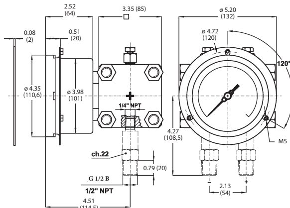
Нижний монтаж (Код A для монтажа), с передним фланцем (Опциональный код F ): DS 4" (100мм)
