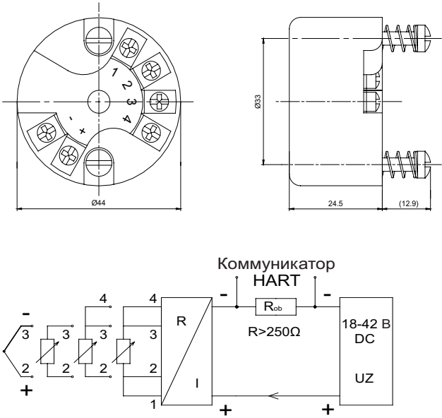
СХЕМА СОЕДИНЕНИЙ
